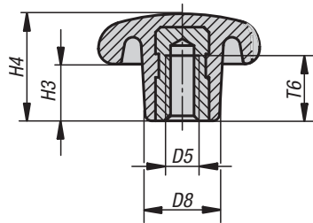
Form K mit Gewindebuchse
